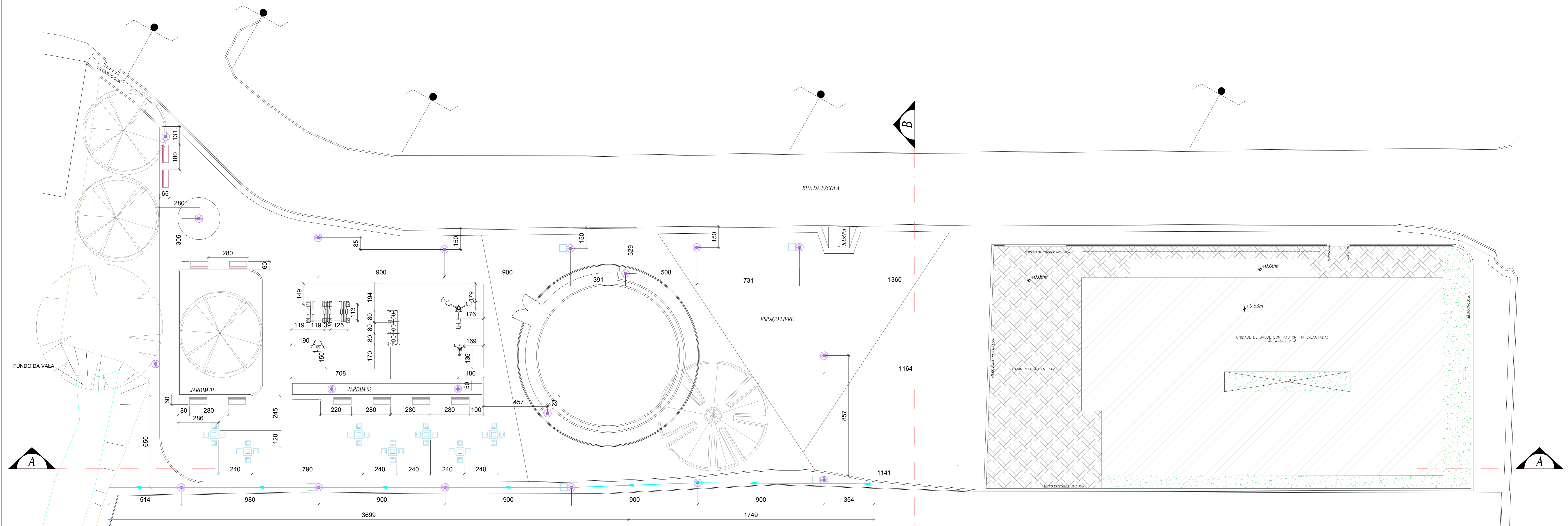
PLANTA DE LOÇÃO DE EQUIPAMENTOS ESC.: 1/100
