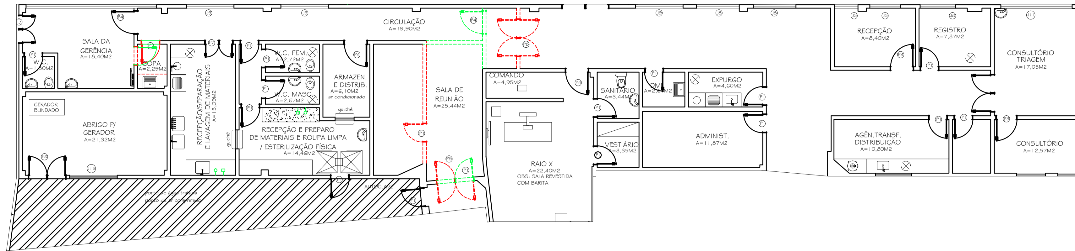
PLANTA BAIXA - ALA 03 ESC.: 1/100
